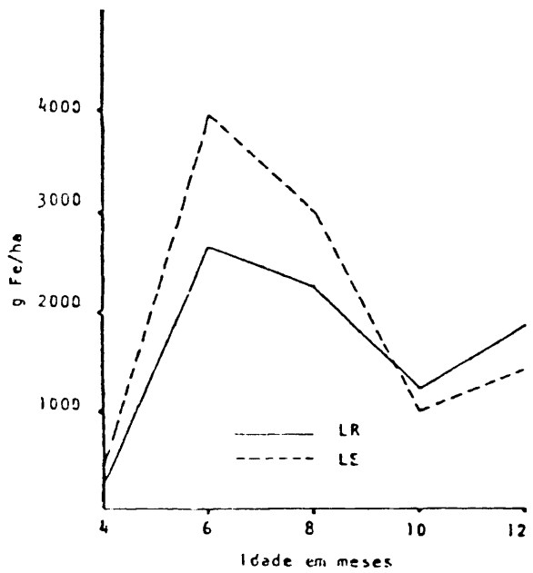
Fig. 7 - Regressões representativas da acumulação de ferro pelos colmos da cana-soca (Y), em função da idade (X) para os solos LR e LE
