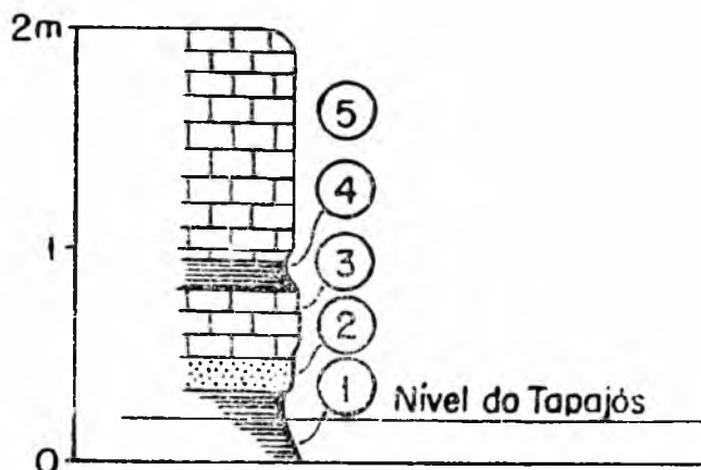
Fig. 3 — Seção na Ponta do Cemitério, Barreiras. 1) Folhelho siltico, azulado; 2) Arenito calcífero, fossilífero; 3) Calcário cinza-claro, fossilífero; 4) Folhelho azulado; 5) Calcário cinza-claro, fossilífero (Foraminíferos).
