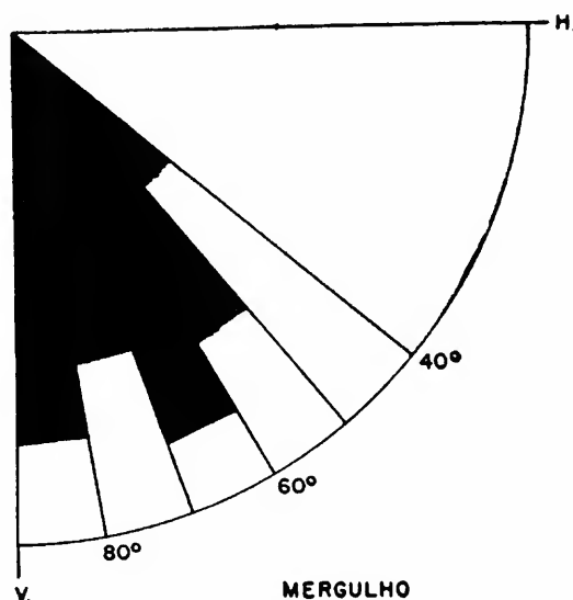
Fig. 7 — Gráfico de variação de mergulho.
