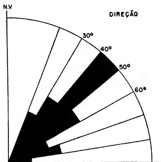
Fig. 6 — Gráfico de variação de direção.
