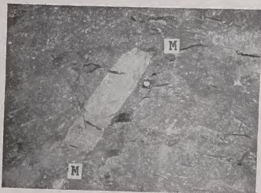
FOTOGRAFIA 4 — Trecho de um dique de aplito róseo com bordos pegmatíticos. Mostra-se falhado por dois planos em que se observou intensa milonitização (m). Pedreira da E. F. Sorocabana.
