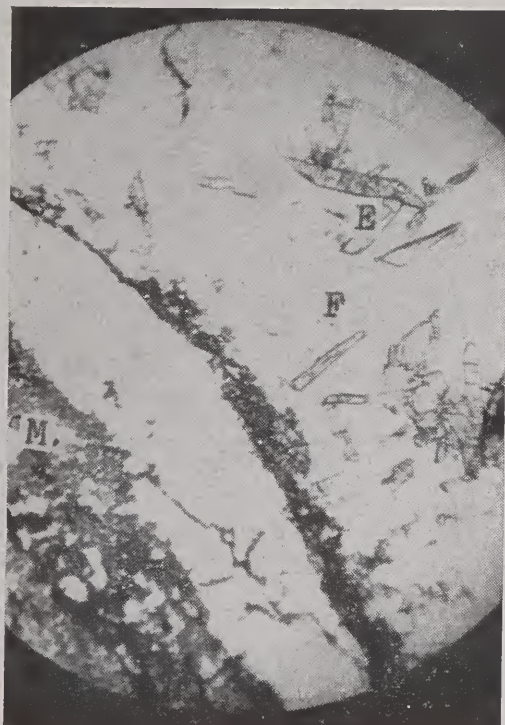
FOTOMICROGRAFIA 14 — Aspecto tomado pelos minerais hidrotermais depositados na capa de um pseudo-dique de milonito. M-milonito. F-fluorita. E-epídoto. Pedr. E. F. Sorocabana. 20X. N. | |.
