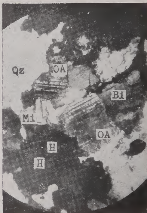
FOTOMICROGRAFIA 11 — Granodiorito. Qz-quartzo. OA-oligoclásio-andesina. Bi-biotita. H-hornblenda. Mi-microclínio. Estrada S. Roque-Ibiuna. 20X. N. +.
