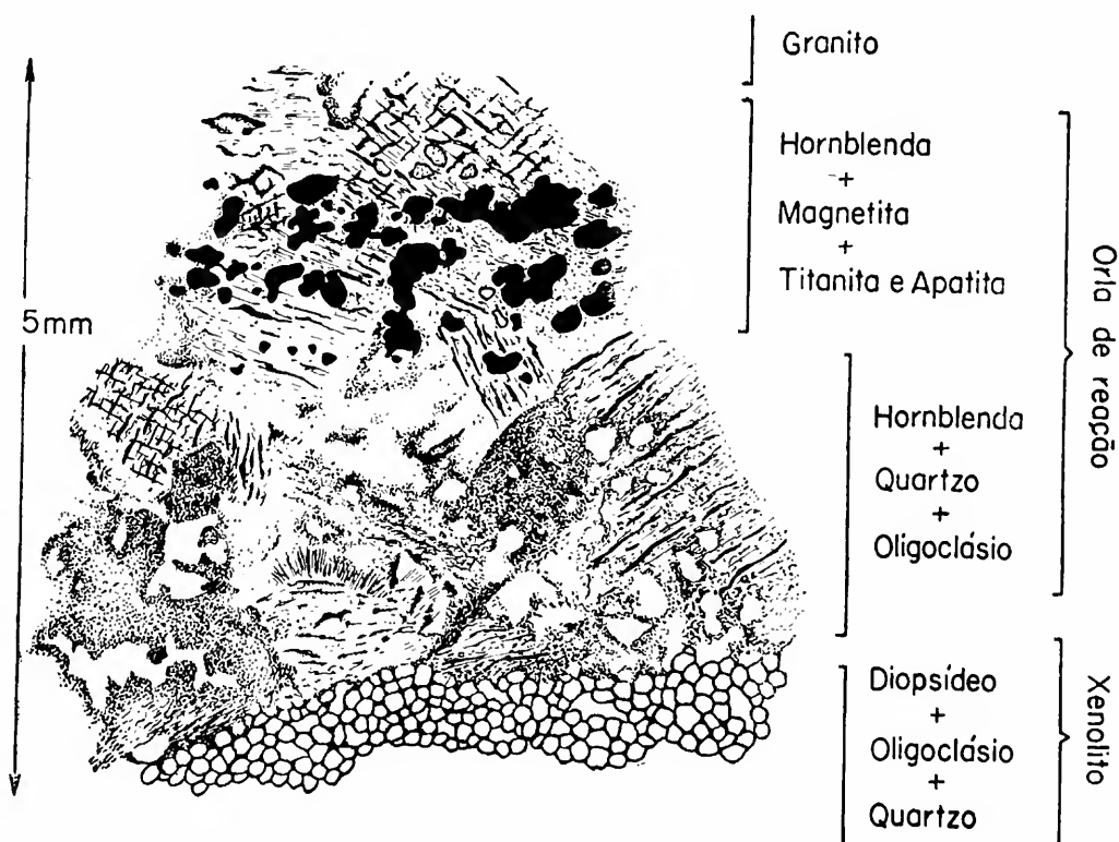
Fig. 10 — Orla de reação do xenólito.
