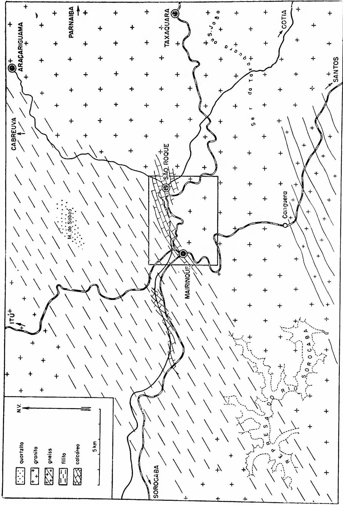
MAPA 1 — Esboço geológico do município de São Roque. Em delimitação retangular a área pesquisada.
