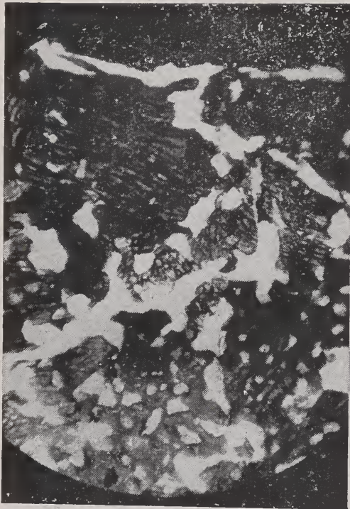
FOTOMICROGRAFIA 1 — Corôa hornblênica do xenólito da foto n.º 5. Hornblenda poiquilítica e inclusões de quartzo e oligoclásio. 35X. N. | |.
