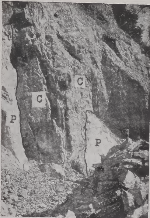
FOTOGRAFIA 2 — Diques de pegmatito (p) caulinizado, concordante com o acamamento vertical do calcário metamórfico (c). Pedreira Sta. Marina.
