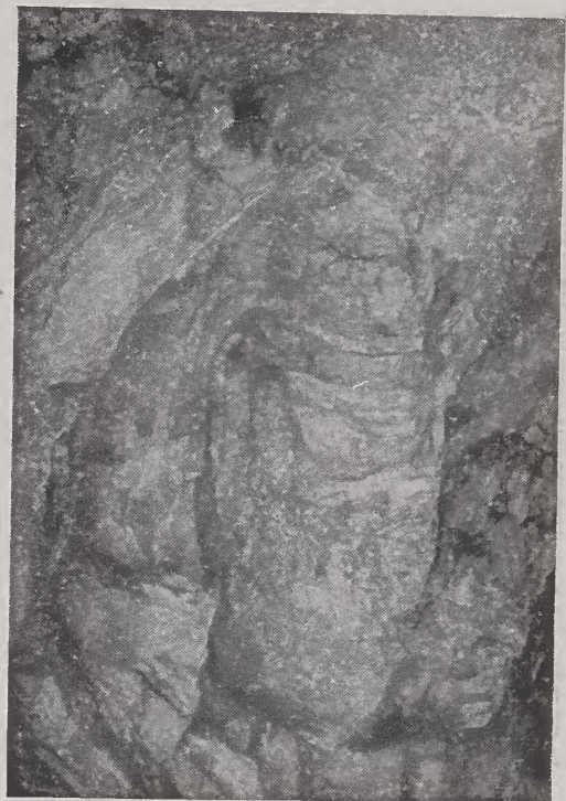
FOTOGRAFIA 3 — Calcário metamórfico intensamente dobrado e plicado nas imediações do contacto com o batolito. Corte da E. F. Sorocabana à altura da bifurcação com a variante para a pedreira da mesma Companhia.
