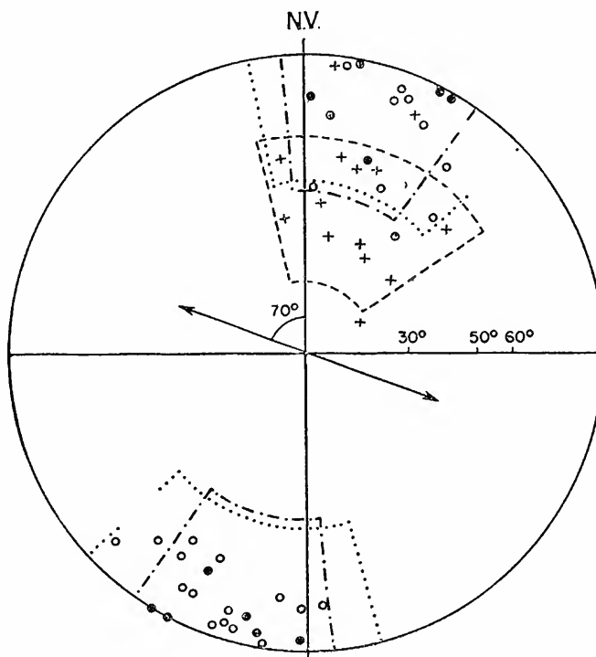
Fig. 4 — Projeção "igual área" dos planos de diques na pedreira E.F.S.
