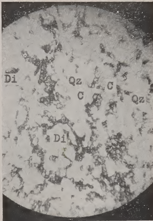
FOTOMICROGRAFIA 16 — Um tipo de camada quartzosa em calcário metamórfico relativamente próximo de contactos. Calcita (C), quartzo (Qz) e diopsídio (Di). Rua da cidade de São Roque. 35X. Nícois | |.
