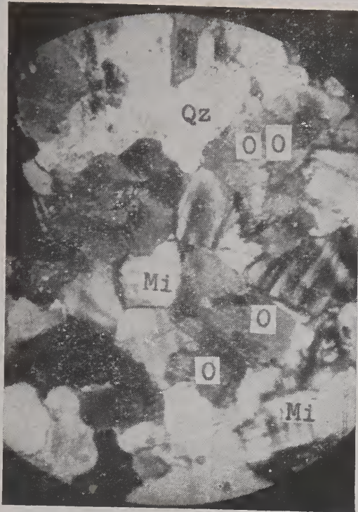
FOTOMICROGRAFIA 12 — Aplito róseo. Nota-se a textura aplítica formada pelos grãos xenomórficos de quartzo (Qz), oligoclásio (O) e microclínio (Mi). Pedr. E. F. Sorocabana. 20X. N. +.
