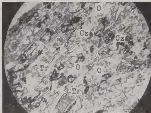
FOTOMICROGRAFIA 15 — Hornfels. Tremolitas (Tr) alongadas e orientadas, aparentando corrosão. Clinozoisita (Cz) em grãos de alto relevo e oligoclásio (O) formando a massa restante. Pedr. E. F. Sorocabana. 20X. N. | |.
