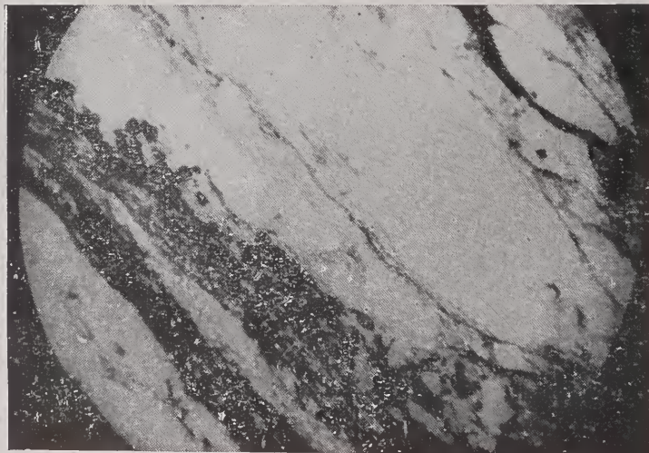
FOTOMICROGRAFIA 2 — Xenólito da foto n.º 5. Formado principalmente por diopsídio (mineral em relêvo), quartzo e oligoclásio. 35X. N. | |.
