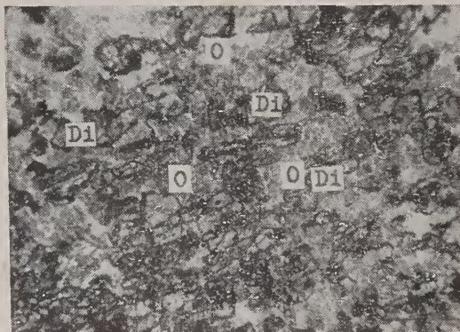
FOTOMICROGRAFIA 17 — Hornfels. Diopsídio (Di) em grãos mostrando clivagens regularmente orientadas em um meio formado exclusivamente por oligoclásio (O). E. F. Sorocabana. 35. N. | |.
