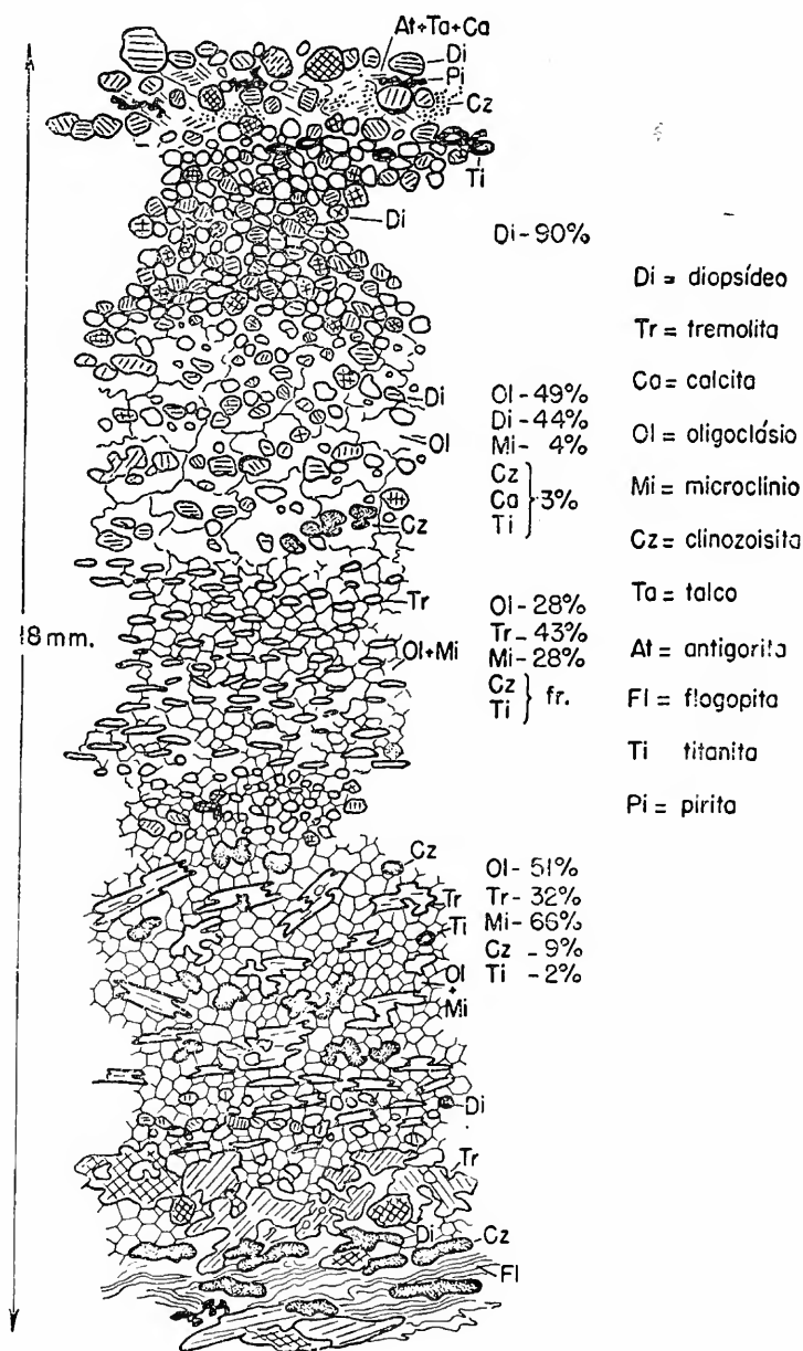
Fig. 11 — Desenho esquemático de lâmina de "hornfels".
