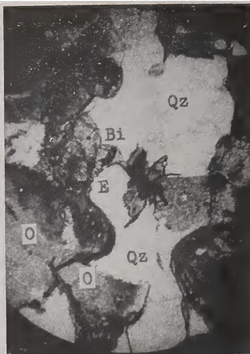
FOTOMICROGRAFIA 9 — Granodiorito Qz-quartzo. O-oligoclásio. Bi-biotita. E-epidoto. E. F. Mairinque-Santos. 20X. N. | |.
