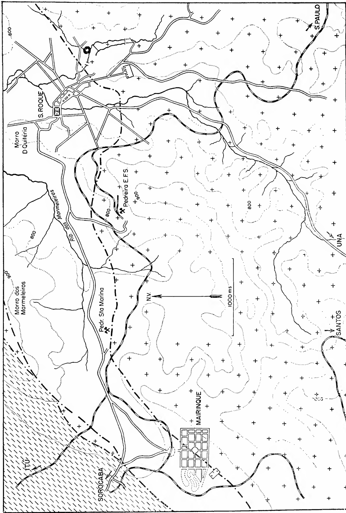
MAPA 2 — Delimitação das formações geológicas na área estudada entre Mairinque e S. Roque.
