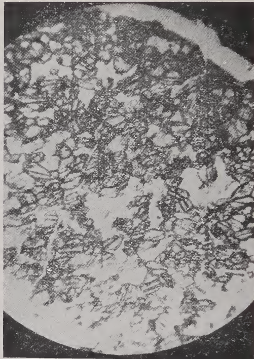
FOTOMICROGRAFIA 2 — Xenólito da foto n.º 5. Formado principalmente por diopsídio (mineral em relêvo), quartzo e oligoclásio. 35X. N. | |.
