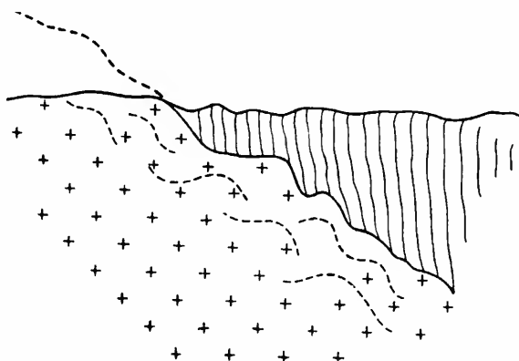
Fig. 3 — Tipo de contacto entre encaixantes e intrusivas, admitido para as ocorrências de São Roque. Em linhas pontilhadas, as direções de mergulho das estruturas fluidais no batolito.
