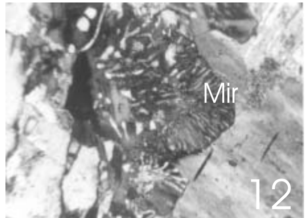
Foto 12. Texturas de intercrescimento mirmequitico caracterizando a atuação de processos de dissolução e transferência de massa durante os estágios tardios da deformação e metamorfismo de baixa temperatura a que as rochas foram submetidas. Mir - mirmequita, aumento de 30X.
