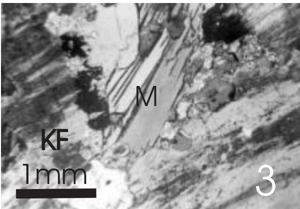
Foto 3. A geração de muscovita resulta da transformação do microclínio. Aumento de 30 X. M - muscovita, KF - microclínio.
