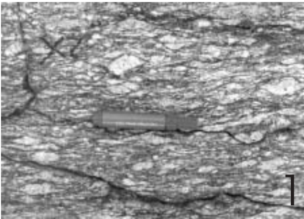
Foto 1. Aspecto textural do augen gnaiss granítico da Serra de São Fernando, caracterizado por fenocristais estirados de K-feldspato de até 5 cm.
