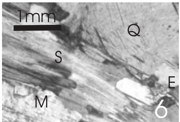
Foto 6. Intensa milonitização nas rochas originais possibilita a formação de sillimanita em processos de metamorfismo e transferência de massa de alta temperatura. Aumento de 30 X. S - sillimanita, M - muscovita, Q - quartzo, E - epidoto.
