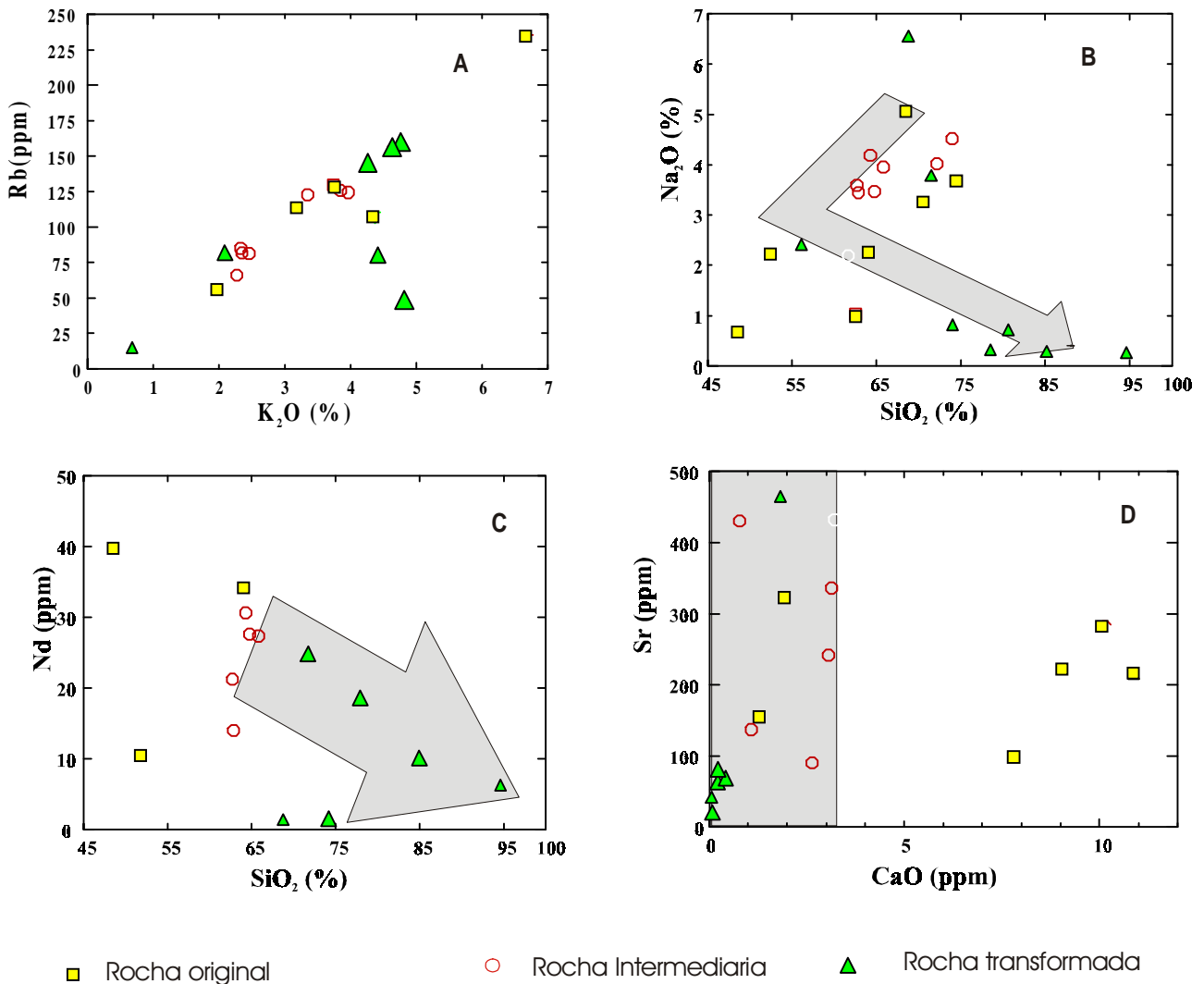
Figura 2. Comportamento dos elementos maiores e traços durante o processo de transformação de rochas. A) Rb x K_2O ; B) SiO_2 x Na_2O ; C) SiO_2 x Nd; D) Sr x CaO. Setas indicam o comportamento dos elementos de acordo com o aumento da deformação e transformação das rochas.
