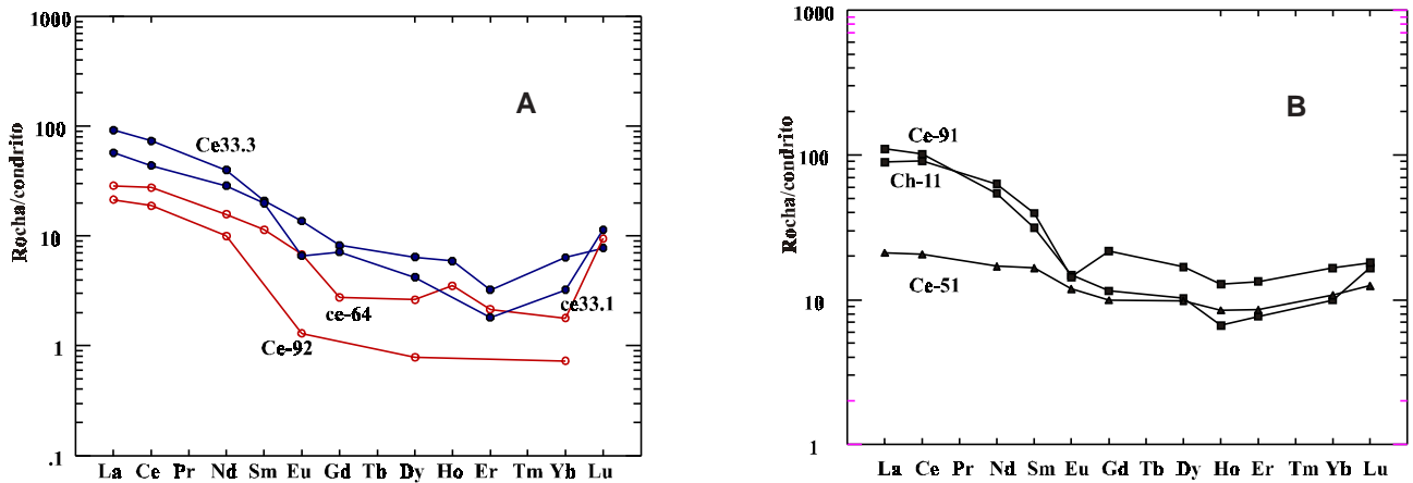
Figura 3. Padrões de Elementos Terras Raras para as rochas estudadas. A) Augen gnaiss, muscovita xisto e muscovita quartzito; B) tonalitos e biotita xistos.
