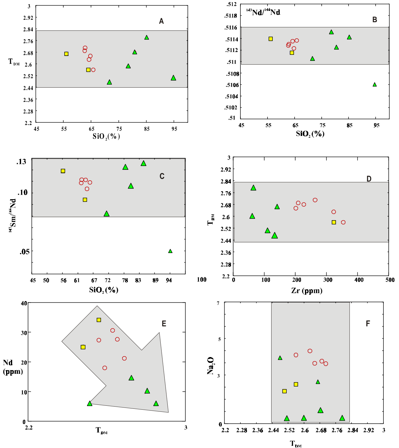
Figura 5. Relações entre os isótopos de Nd e a sua variação durante os processos de milonitização. Setas indicam o comportamento dos elementos de acordo com o aumento da deformação e transformação das rochas. Também é mostrado o campo de superposição entre os valores de idade modelo T_{DM} e razões isotópicas das rochas originais e transformadas. A) T_{DM} x SiO_2 ; B) ^{143}Nd/^{144}Nd x SiO_2 ; C) ^{147}Sm/^{144}Nd x SiO_2 ; D) T_{DM} x Zr; E) Nd x T_{DM} ; F) Na_2O x T_{DM} .
