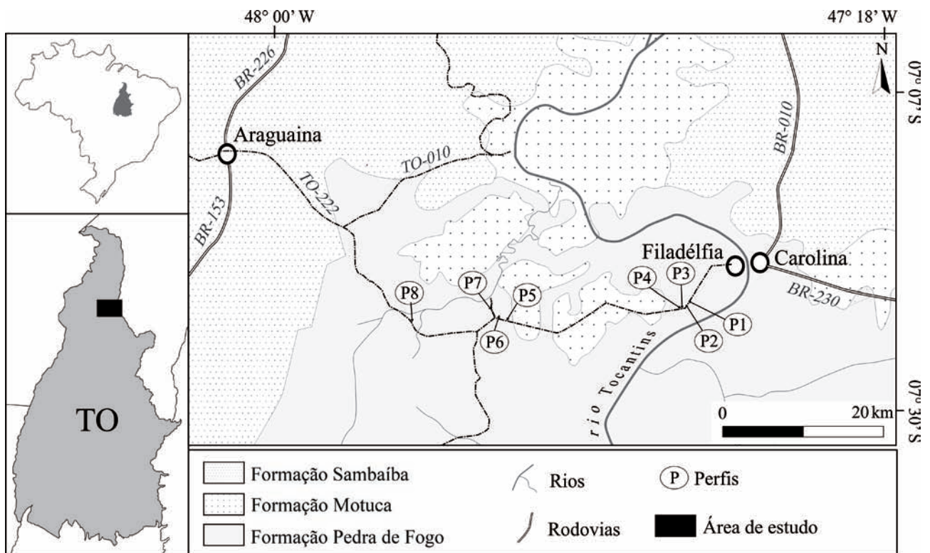
Figura 1. Localização e geologia da região de Filadélfia, Estado do Tocantins.
