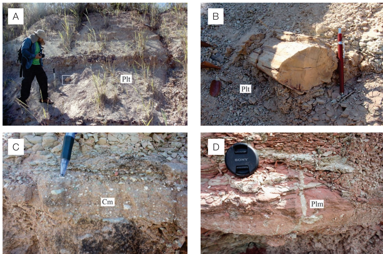
Figura 5. (A) Camadas tabulares centimétricas de arenito fino intercaladas com pacotes decimétricos de pelito cinza laminado com troncos fósseis (Plt); (B) detalhe do tronco silicificado imerso no pelito; (C) camada de arenito fino a siltico, com clastos de argila e silex dispersos caoticamente (Cm); (D) detalhe do pelito laminado a maciço (Plm).
