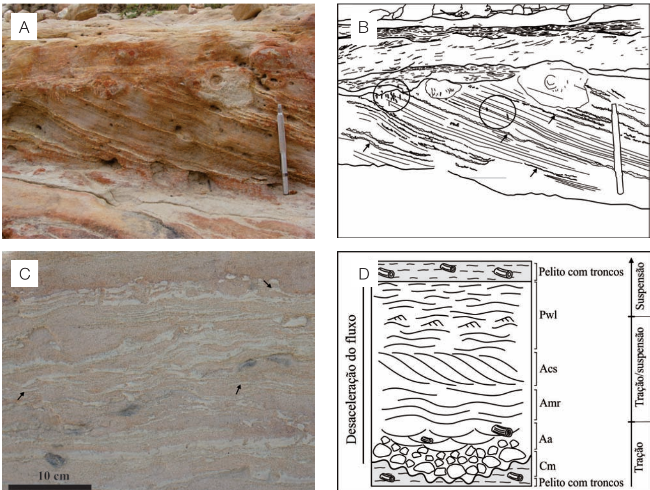
Figura 11. Sucessão de estruturas representativas da parte superior do depósito de inundito. (A e B) Arenito fino a médio com estratificação cruzada tabular a sigmoidal e foresets recobertos por mud drapes descontínuos e irregulares (setas). Observar também cristais centimétricos de evaporitos (círculo); (C) ritmito arenito/pelito com acamamento wavy/linsen e eventuais laminações cruzadas com rip-up clasts e curled flakes (setas); (D) perfil esquemático mostrando a sucessão de estruturas que indicam desaceleração do regime de fluxo, interpretada como depósito de inundito.
