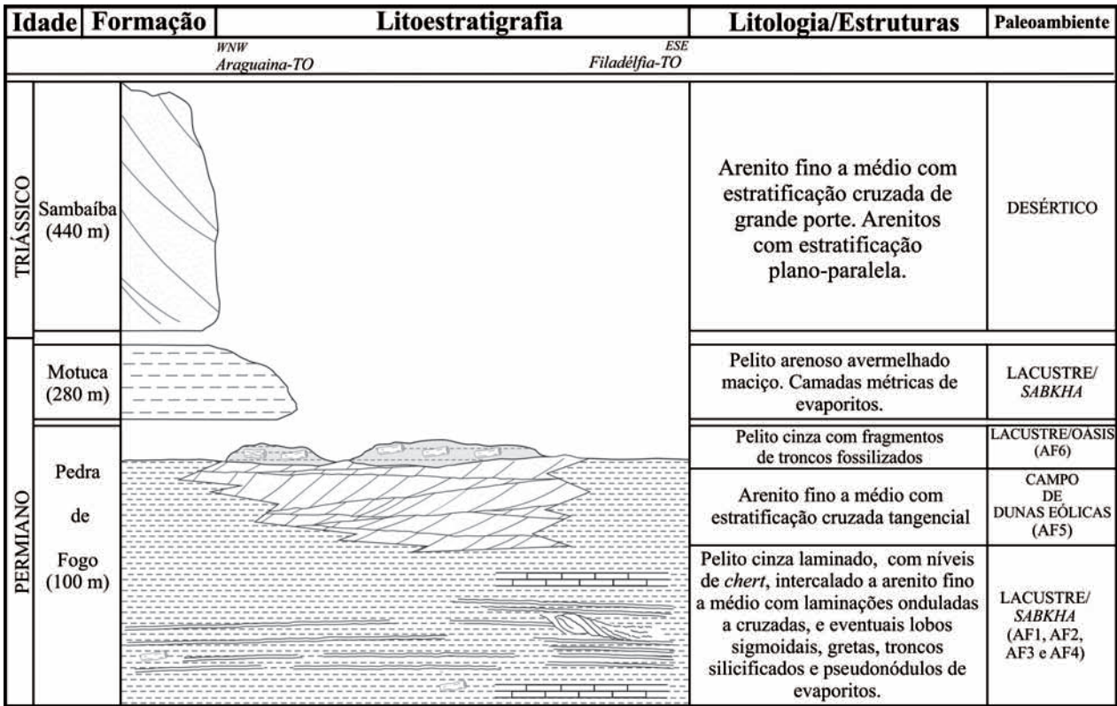
Figura 2. Coluna litoestratigráfica da região de Filadélfia, TO, com descrição das principais litologias e ambientes deposicionais.
