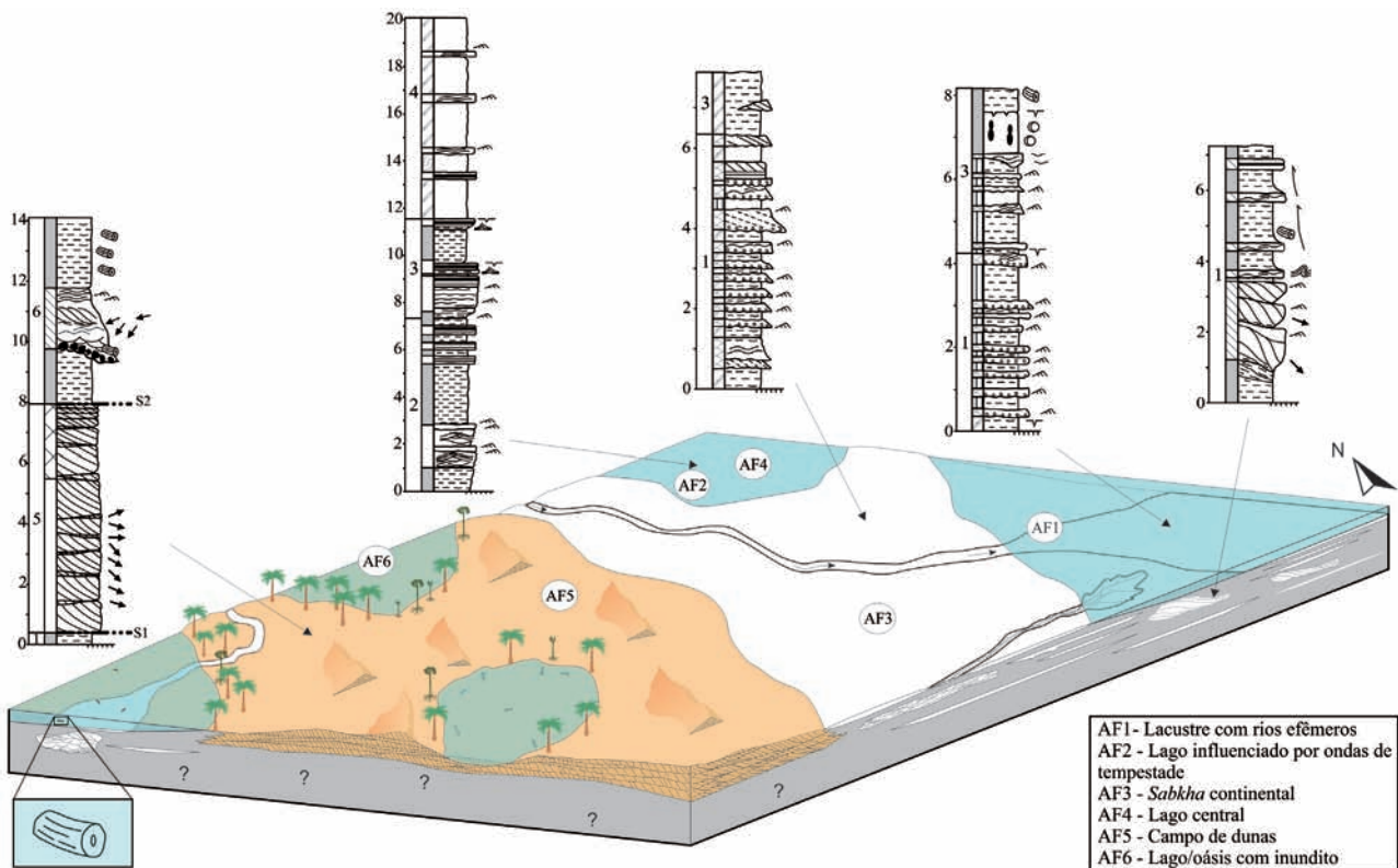
Figura 13. Modelo deposicional da parte superior da Formação Pedra de Fogo na região de Filadélfia, TO.
